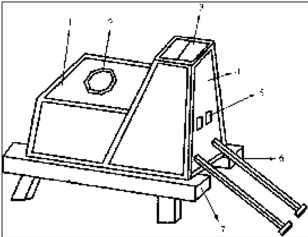
据《武经总要》复原之行炉示意图
