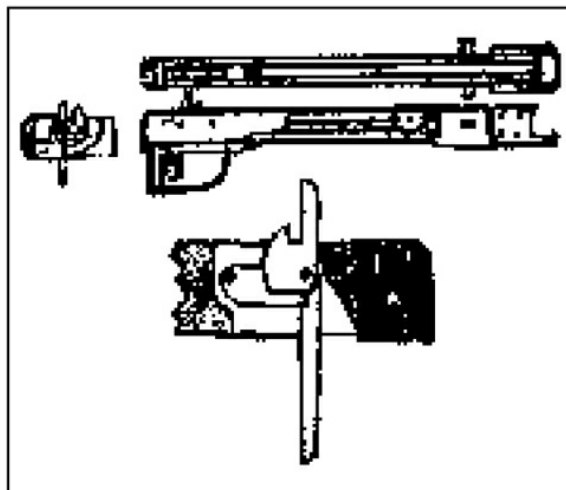
战国弩机结构
